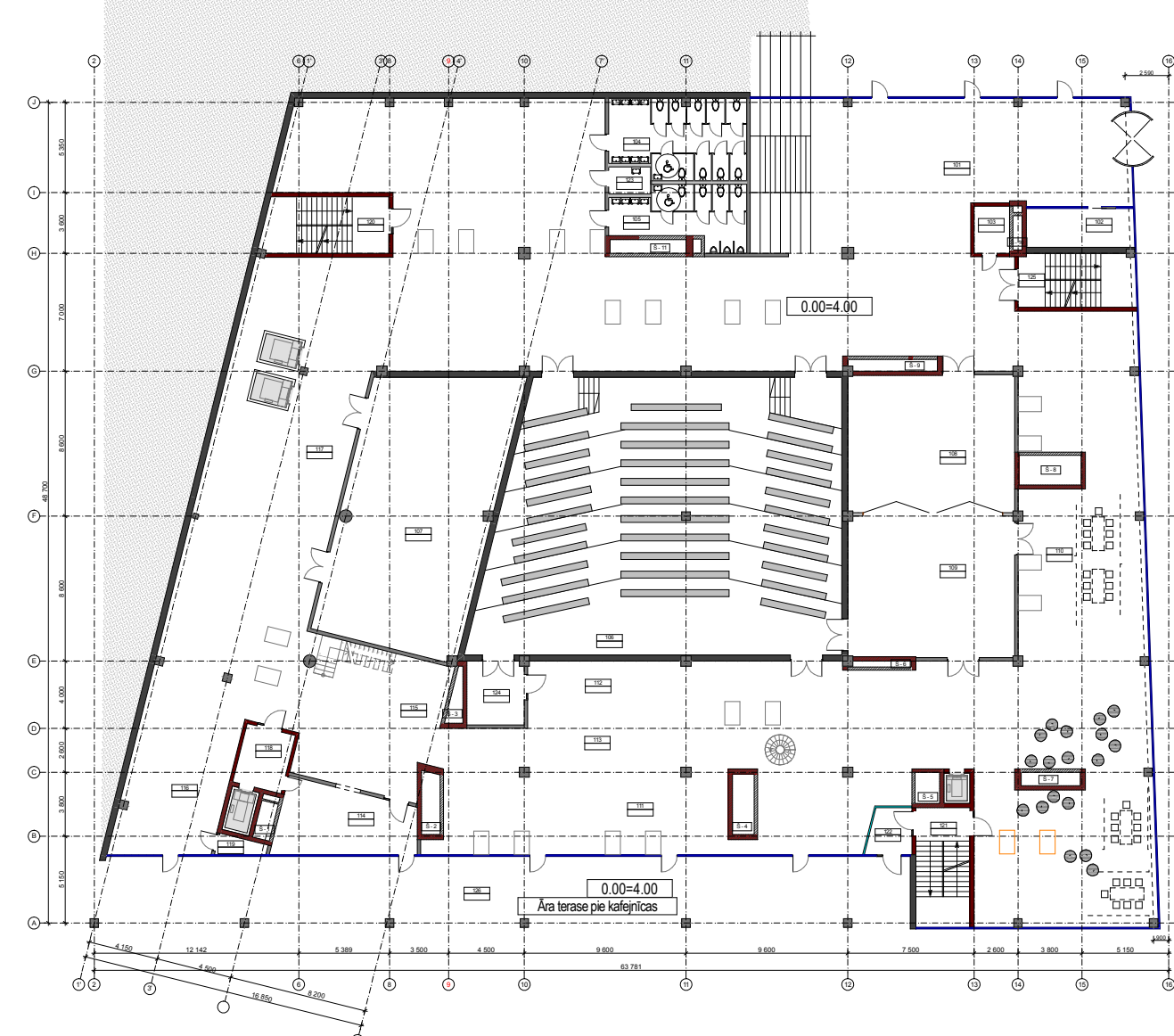
1. STĀVS
