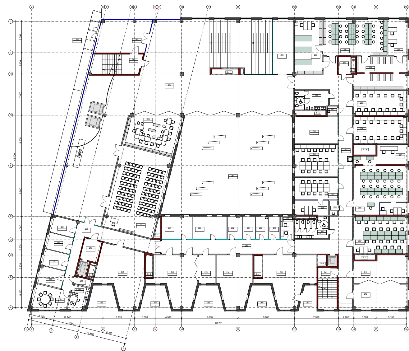
2. STĀVS
